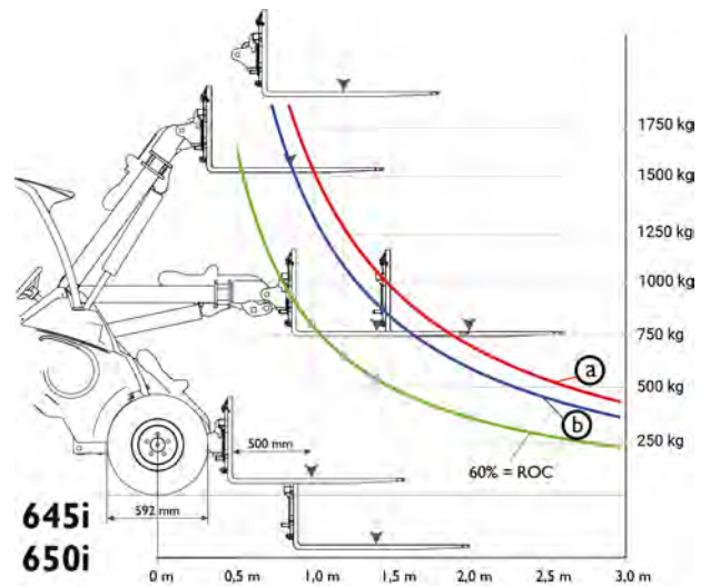
Diagrama de cargas de 645i/650i
